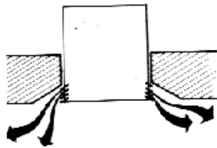
Detalhe em planta: Ar-condicionado na parede
